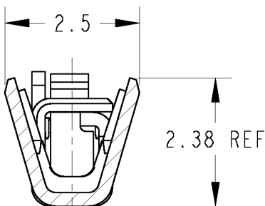
断面 B-B
