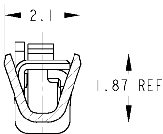
断面 A-A
